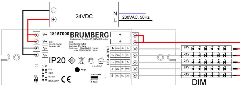
Anschlussbild 1: Für den Anschluss von 1 farbigen LEDs oder "dim to warm LEDs"
